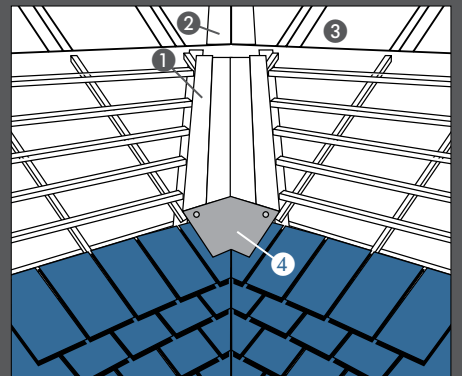
Gesloten kielgoot
