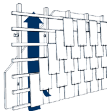
dekking met open voeg
